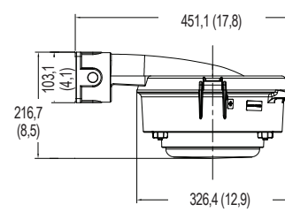
Montage mural — Diffuseur
