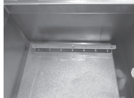
Support pour rail sans plaque de montage.
