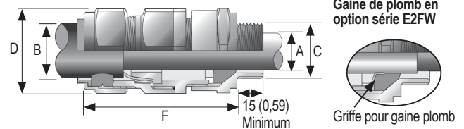
Dimensions en millimètres (pouces)
