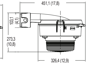
Montage mural — Réfracteur
